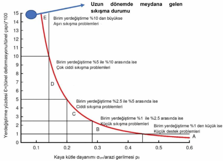
Şekil 13. Desteksiz tünellerde birim yerdeğışirmeye bağılı olarak meydana gelen sıkışma problemlerinin derecesini tahmin abağı (Hoek ve Marinos, 2000).
